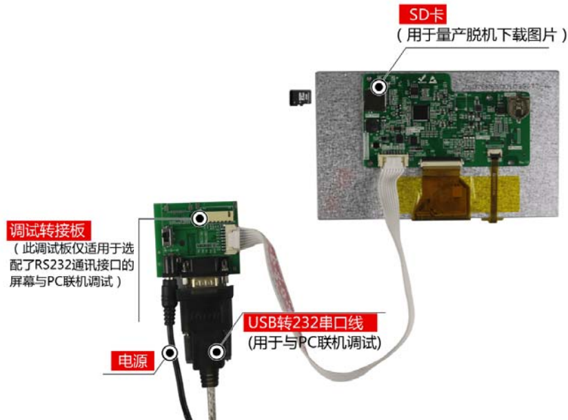
图 1-4 调试工具图
